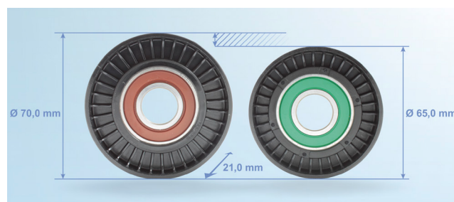
Εικόνα 2: Τροχαλία παρέκκλισης 532 0404 30 για αυτοκίνητα με κινητήρα βενζίνης (αριστερά) και τροχαλία παρέκκλισης 532 0406 30 για αυτοκίνητα με κινητήρες πετρελαίου (δεξιά)
