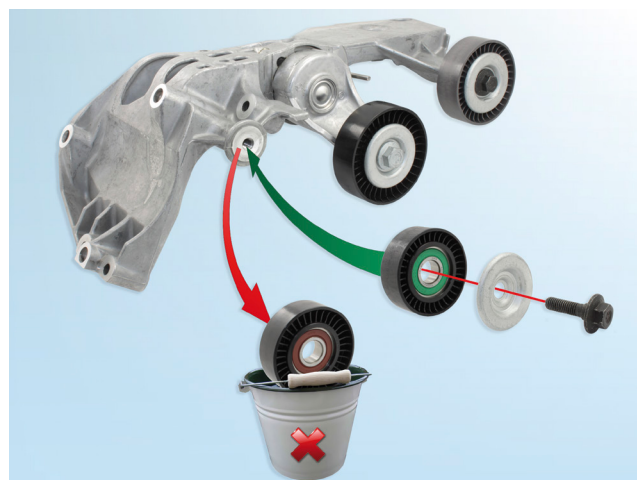
Εικόνα 1: μονάδα τάνυσης 534 0243 10
