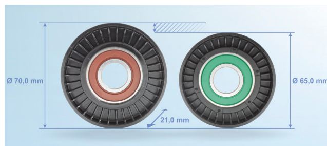
Figur 2: Venderulle 532 0404 30 til kjøretøy med bensinmotor (venstre) og venderulle 532 0406 30 til kjøretøy med dieselmotor (høyre)
