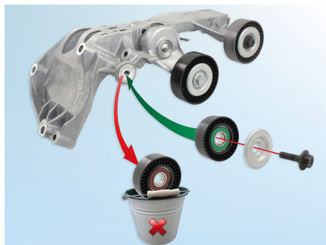
Рисунок 1: Натяжной узел 534 0243 10
