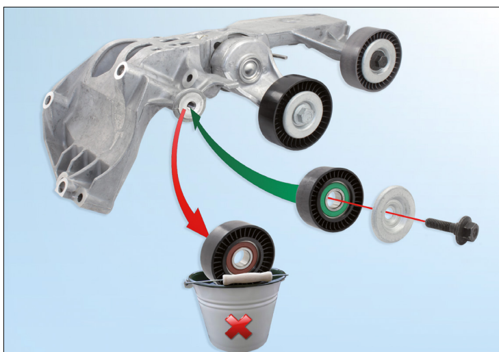
Obrázok 1: Napínacia jednotka 534 0243 10
