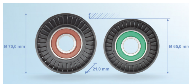
Bild 2: Styrrulle 532 0404 30 till fordon med bensenmotor (vänster) och styrrulle 532 0406 30 till fordon med dieselmotor (höger)
