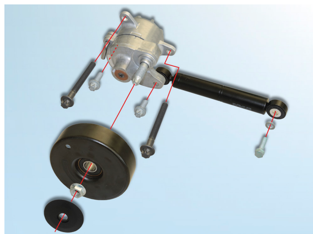
Εικόνα 1: 533 0116 10 – σετ επισκευής INA για το σύστημα κίνησης συμπεριλαμβανομένων και των κοχλιών στερέωσης
