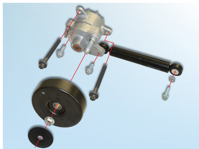
Figur 1: 533 0116 10 – reparasjonskita INA pro pohon agregátů včetně upevňovacích šroubů
