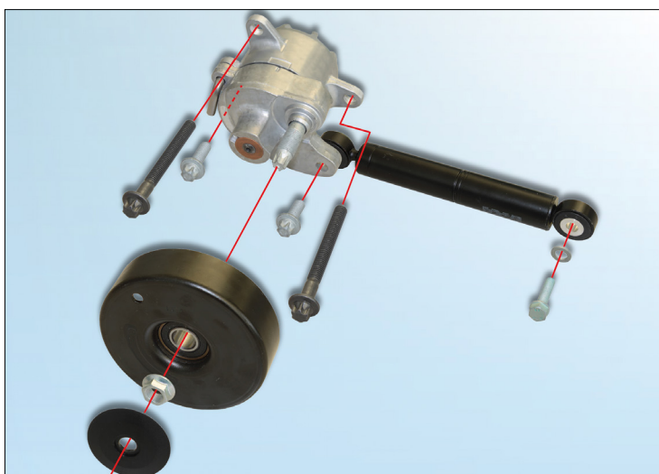
Slika 1: 533 0116 10 – INA garnitura proizvajalca INA za popravilo sklopa pogona s priloženimi privojnimi vijaki
