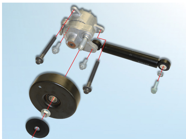
Bild 1: 533 0116 10 - reparationssats INA för hjälppaggregatdrivning, inkl. fästsruvar
