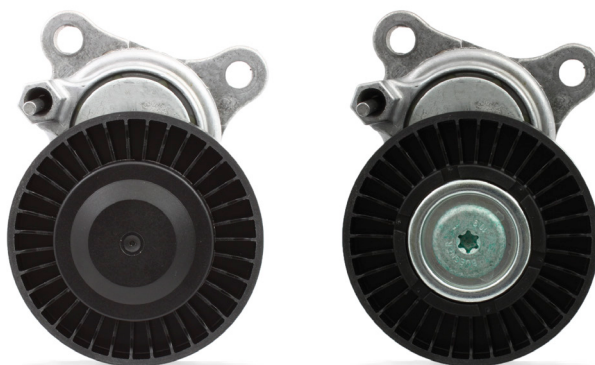
Рисунок 1: Предыдущая конструкция (слева) и новая конструкция (справа)
