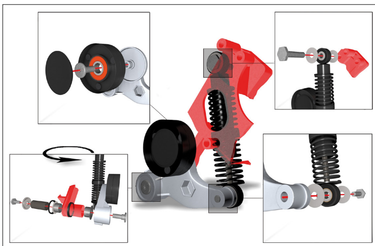
Slika 2: Pregled pričvršnih dijelova
