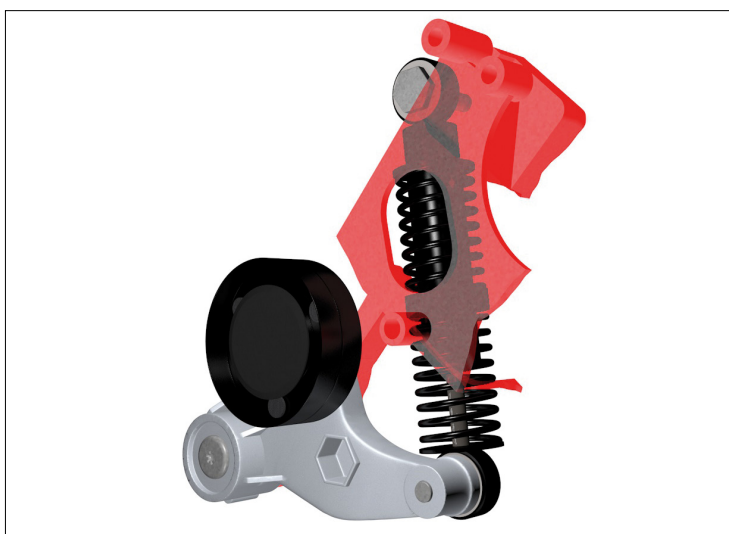
Slika 1: Kompletirana jedinica natezača
