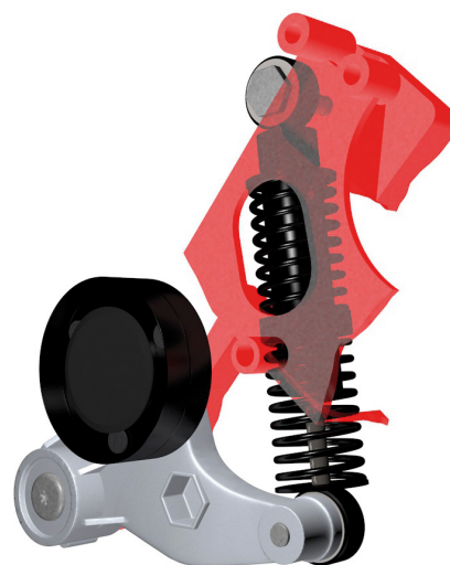
Рисунок 1: Натяжной модуль в сборе
