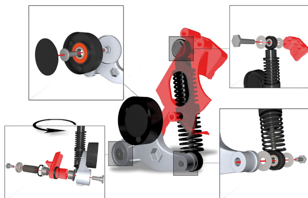
Рисунок 2: Обзор крепежных частей
