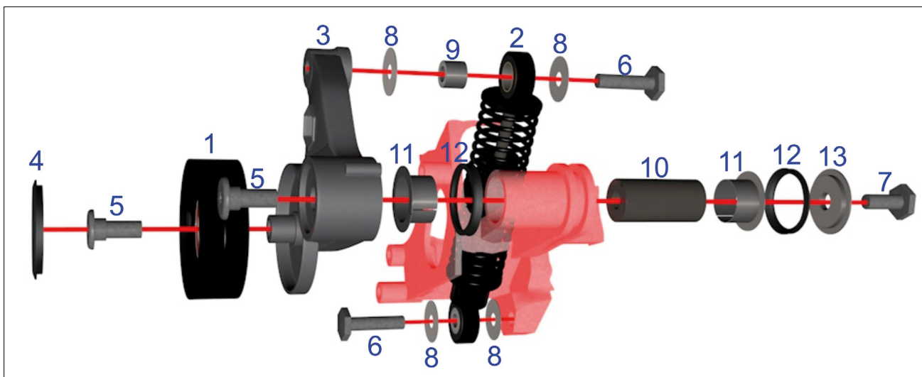
Рисунок 3: Ремкомплект INA 533 0118 10 для натяжного узла
