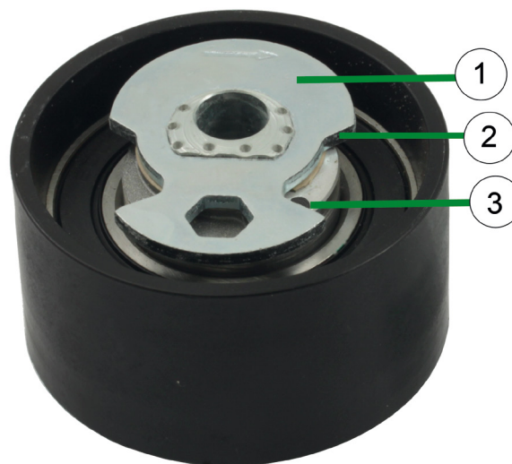
Kuva 1: 531 0504 10 – puoliautomaattinen kiristinpyörä
