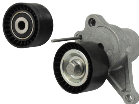
Figur 2: Spennrulle og venderulle i plast
