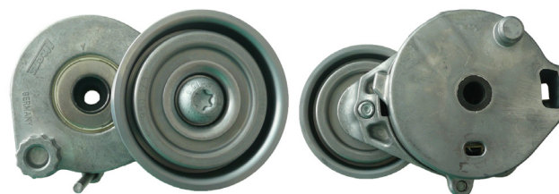
Рисунок 2: Новая конструкция
