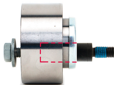
Рисунок 4: Натяжной ролик с втулкой и крепежным болтом в установленном положении
