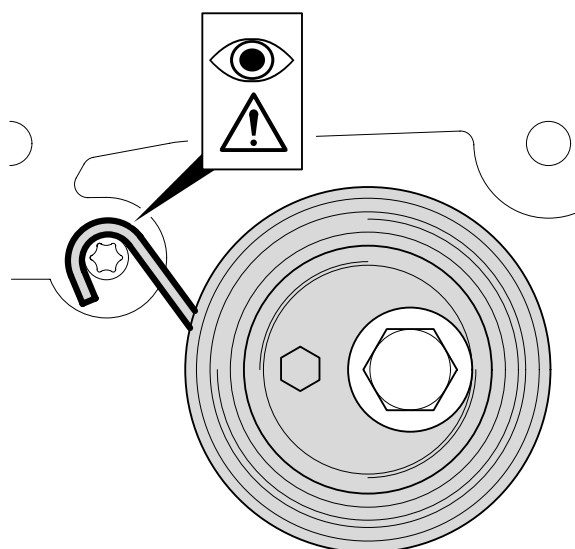
Obrázek 1: Správná montážní poloha pružiny na aretačním čepu
