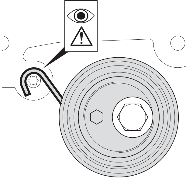
Resim 1: Yayın ankraj civatasına doğru şekilde takılması
