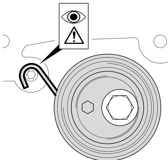
Зображення 1: Правильна фіксація пружини анкерним гвинтом
