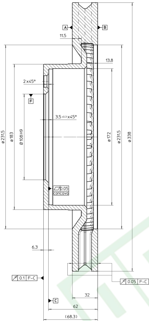
Sezione A-A
