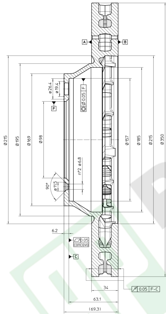
Sez. A-A
