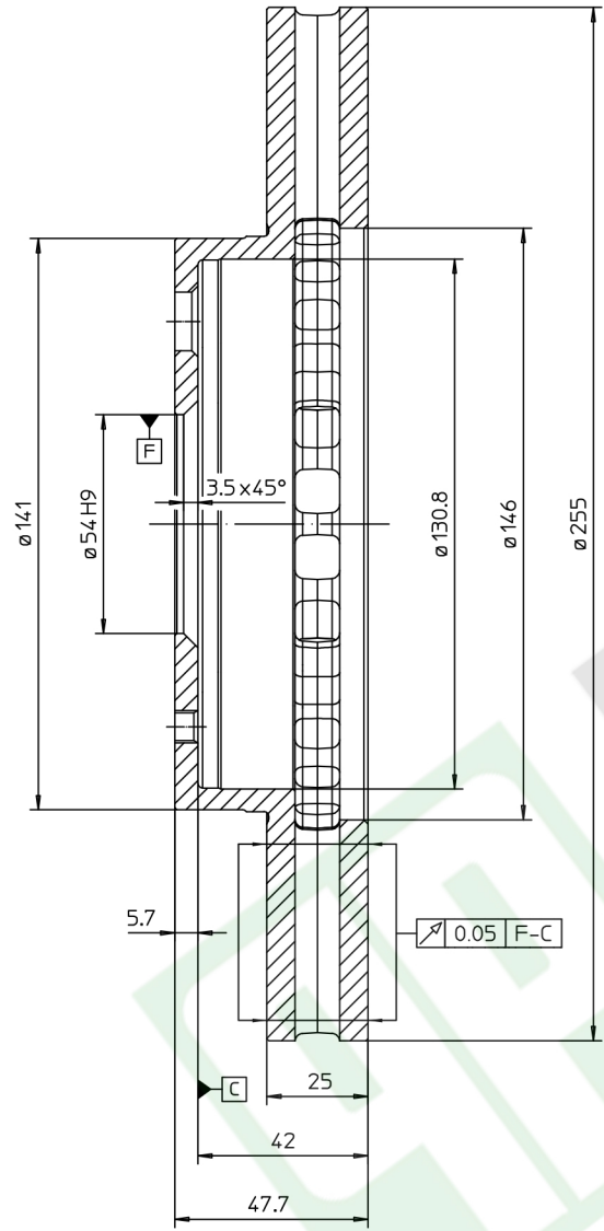
Sezione A-A
