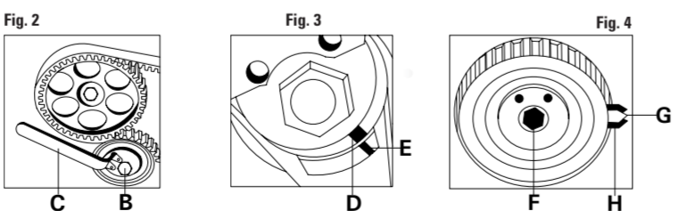
FIGURA 2 Allentare il bullone di bloccaggio B e ruotare in senso orario il tendicinghia utilizzando la chiave C agendo sull'eccentrico di registro. FIGURA 3 Allineare l'indicatore D del tendicinghia con la tacca E, serrare quindi il bullone di bloccaggio B. FIGURA 4 Allentare il bullone di bloccaggio F del tendicinghia e ruotare quest'ultimo in senso orario fino ad allineare l'indicatore G con la zona di controllo H.
