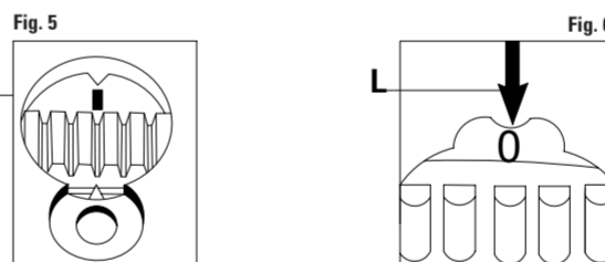
FIGURA 5 Segni di riferimento sul volano: verificare il corretto allineamento delle tacche di fase L. FIGURA 6 Segni di riferimento sul volano: verificare il corretto allineamento delle tacche di fase L.
