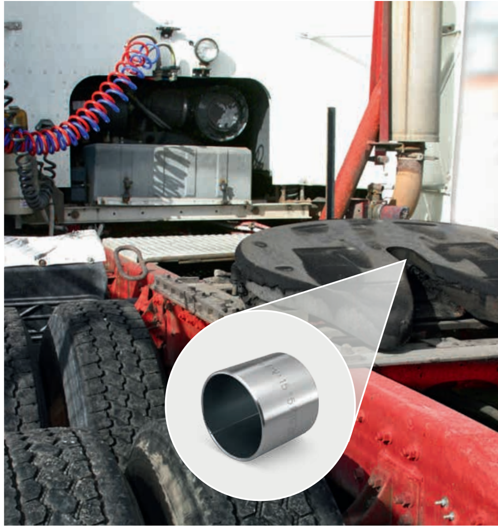
Yarı römork kavramada KS PERMAGLIDE® P10 kaymalı yatak burçları ile yataklama
