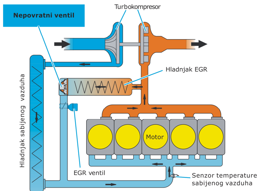
Šema recirkulacije izduvnih gasova sa hlađenjem
