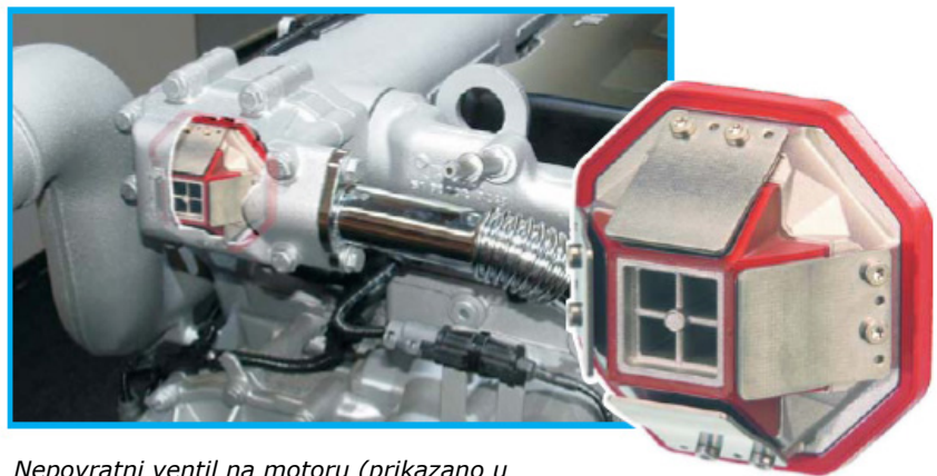
Nepovratni ventil na motoru (prikazano u preseku)
