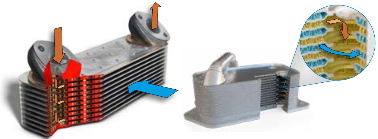
مبرد الزيت بالمركبات التجارية
