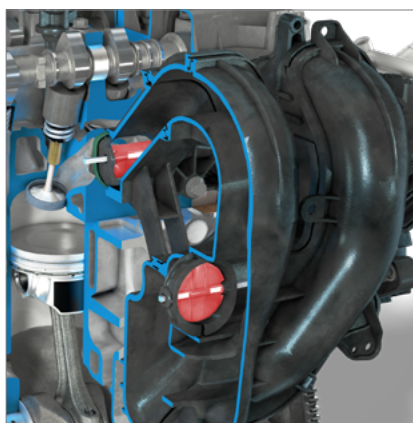
Klapy w kolektorze dolotowym
