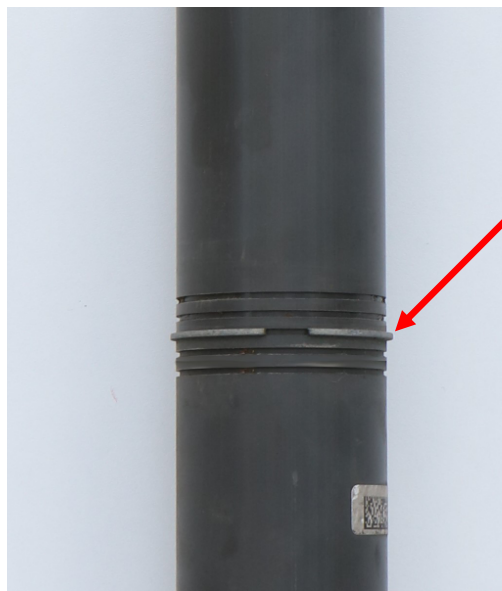
Abb. 5: Sprengring in Nut 3/5 von unten montieren (Targa: 4/5 von unten) Fig. 5: Install the snap ring in groove 3/5 from bottom (Targa: 4/5 from bottom)
