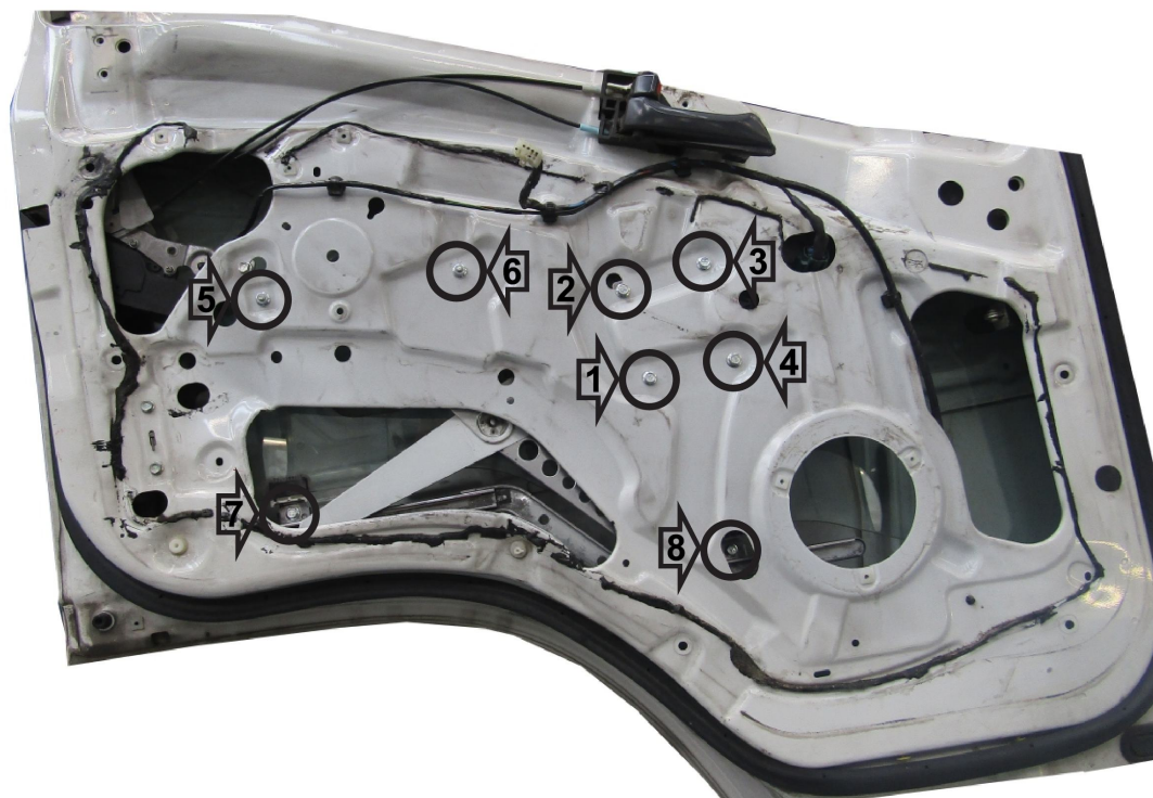
Porta lato sinistro - Left hand side door
