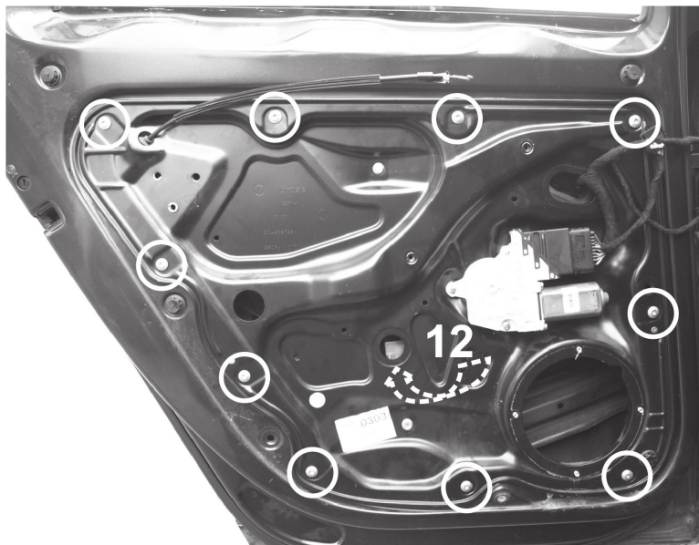
Porta lato sinistro - Left hand side door
