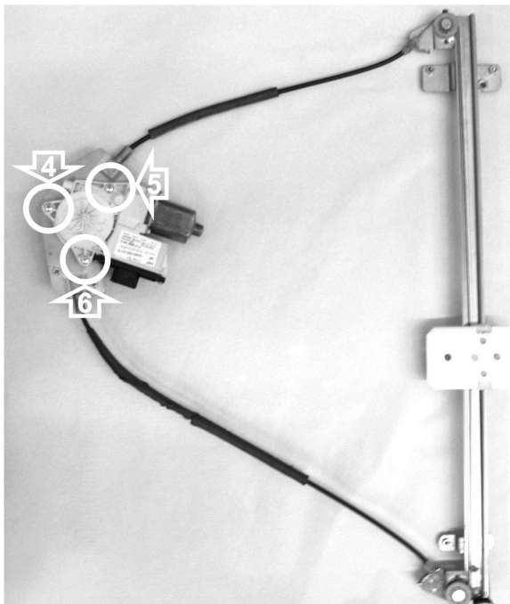
Porta lato sinistra- Left hand side door
