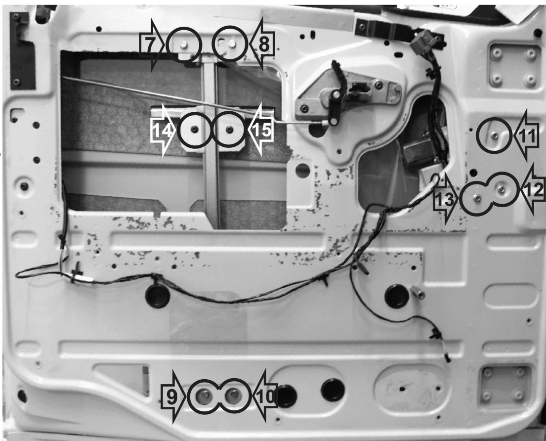
Porta lato sinistro - Left hand side door - Porte latérale gauche - Linken Seitentür
