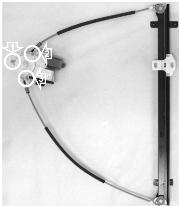
Porta lato sinistra- Left hand side door
