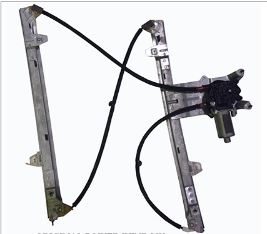
ORIGINAL POWER WINDOW ALZACRISTALLI ELETTRICO ORIGINALE
