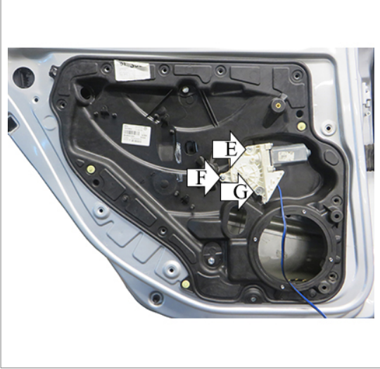
POWER WINDOW LIFTER ALZACRISTALLI ELETTRICO
