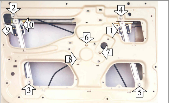
Skoda Felicia - Pick-up (>7/1996)
