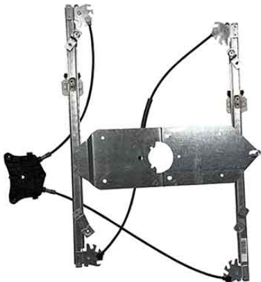
POWER WINDOW LEFT ALZACRISTALLI ELETTRICO SINISTRO
