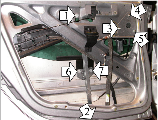
ELECTRIC POWER WINDOW LEFT ALZACRISTALLO ELETTRICO SX
