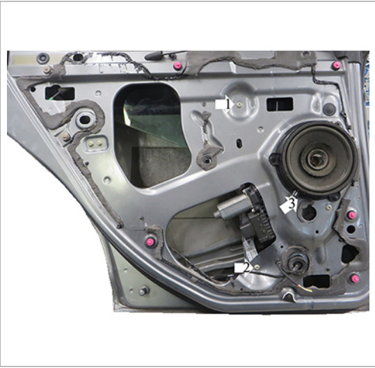
POWER WINDOW LEFT ALZACRISTALLI ELETTRICO SINISTRO
