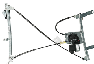
POWER WINDOW LEFT ALZACRISTALLI ELETTRICO SX
