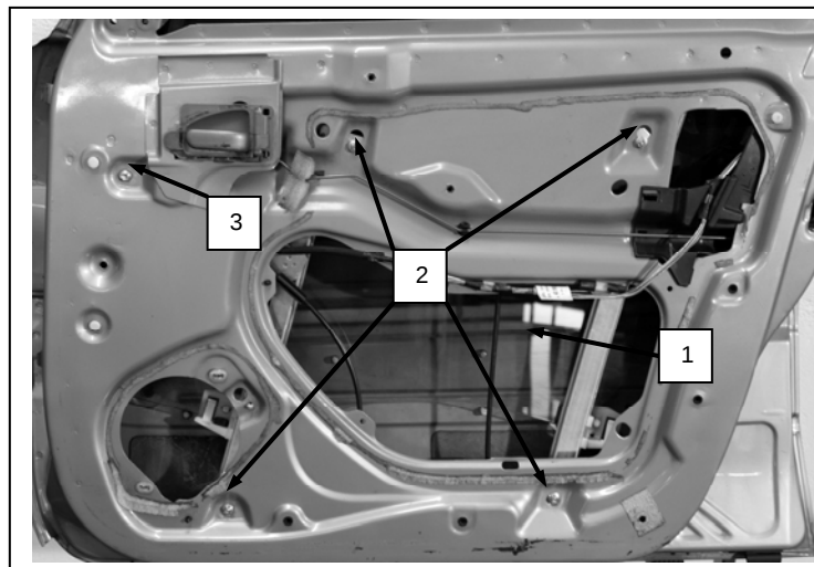
Porta lato destro, Portière avant droite, Right front door, Puerta lado derecho, Vorne rechte Tür, Porta frente dirieta, Sağ on kapi, πόρτα εμπρός δεξιά
