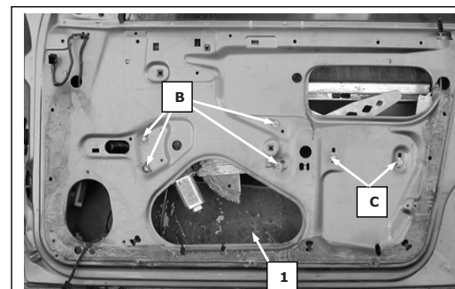
Porta lato destro, Portière avant droite, Right front door, Puerta lado derecho, Vorne rechte Tür, Porta frente dijeta, Sag on kapi, νόρτα εμπρόσθια δεξιά
