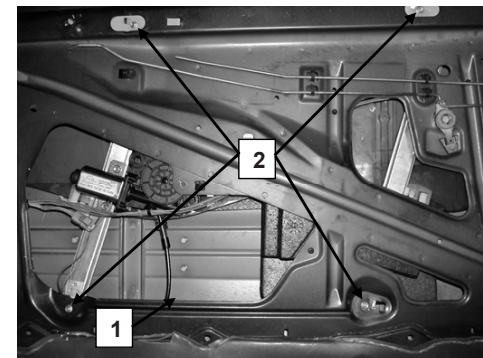
Porta lato destro, Portière avant droite, Right front door, Puerta lado derecho, Vorne rechte Tür, Porta frente dirota, Sag on kapi, πόρτα εμπρός δεξιά
