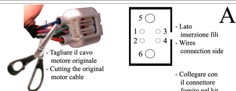
POWER WINDOW LEFT ALZACRISTALLI ELETTRICO SX
