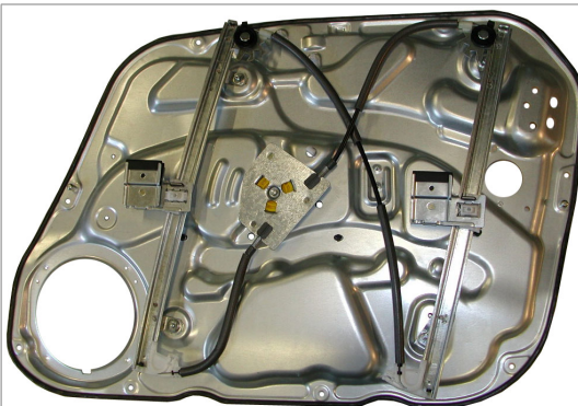
A POWER WINDOW LEFT ALZACRISTALLI ELETTRICO SX
