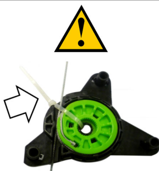
- POSIZIONE INSERIMENTO IN PORTIERA ALZACRISTALLI ELETTRICO. - POWER WINDOW INSTALLATION POSITION INTO THE DOOR.
