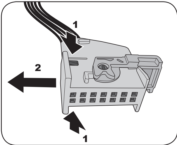
Stecker 14 pin E-Satz connector 14 pin e-kit
