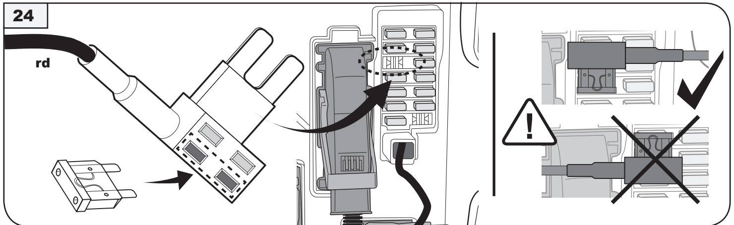
Sicherung 20A → E-Satz rd → Kammer 3 fuse 20A → e-kit rd → fuseslot 3
