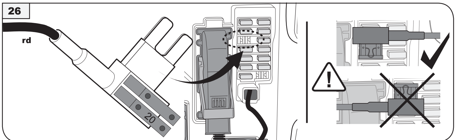
E-Satz rd → Kammer 3 e-kit rd → fuseslot 3
