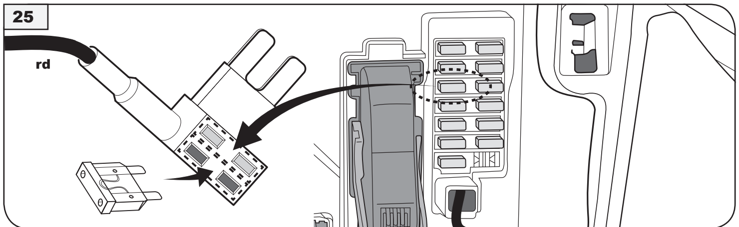
Sicherung 20A → E-Satz fuse 20A → e-kit
