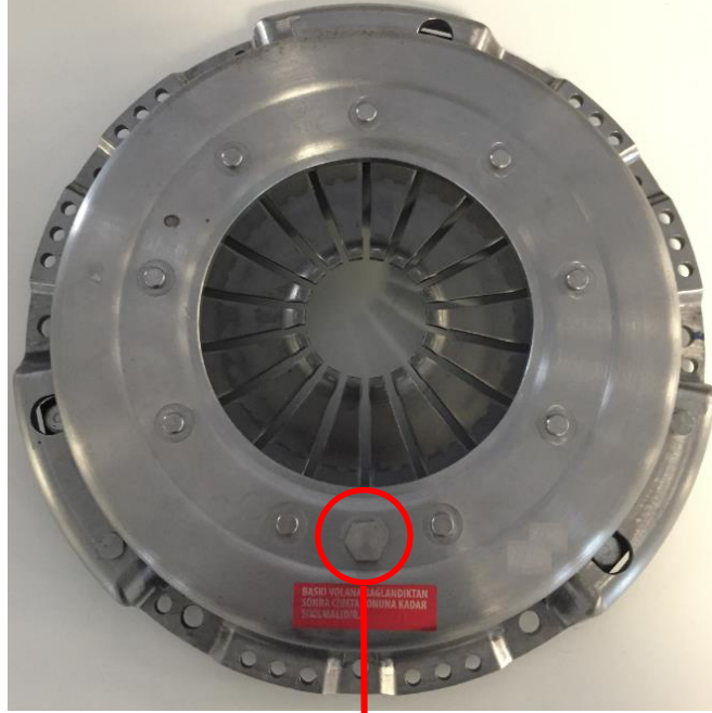
Altı Köşe Başlı Civata (Anahtar Ağzı 13)
