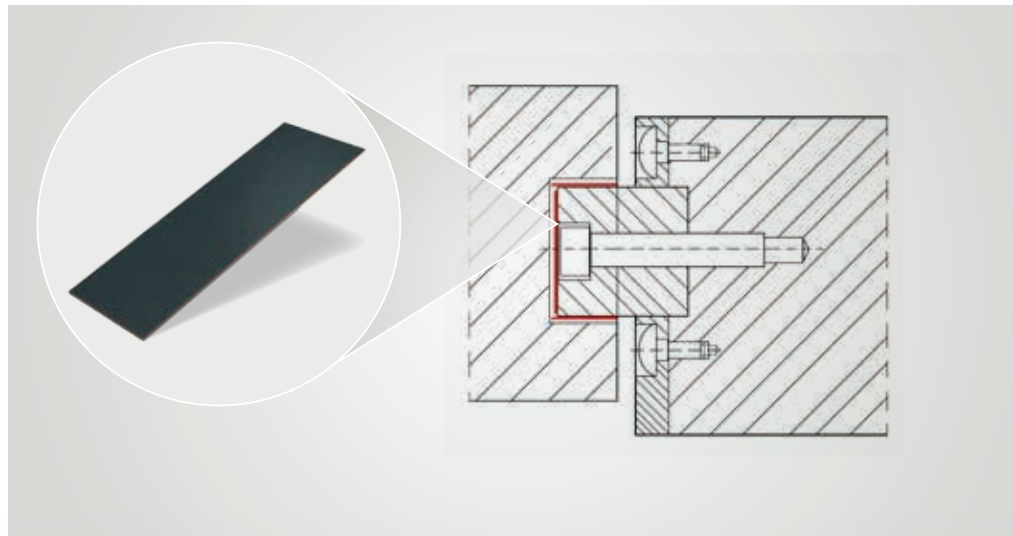
Kayar tezgahların PAS ... P11 yapı türündeki PERMAGLIDE® kaymalı yatak şeritleri ile yataklanması
