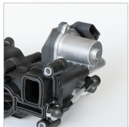
Für einzelne Saugrohre hat Motorservice auch die passenden Anbauteile, wie elektrische Antriebsmodule, im Programm.
