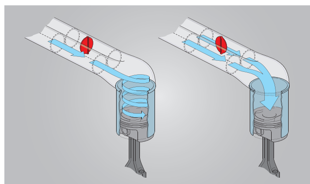
Rys. 1: Klapa zawirowująca: zawirowanie w kierunku osi tłoka po lewej stronie: obciążenie częściowe, klapa zawirowująca zamknięta, silne zawirowanie po prawej stronie: obciążenie pełne, klapa zawirowująca otwarta, wysoki stopień napełnienia
